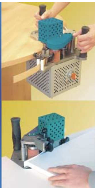
Обрезной станок для кромок ПВХ и АБС до 3 мм
